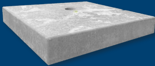
Steini 80 RAF - vörundur. S080 175 kg. 80x80x12 cm.
