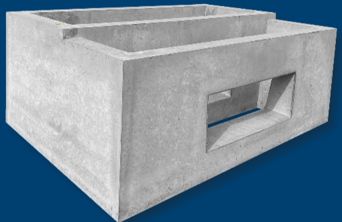
Kempower Triple - vörundur. S051 1.560 kg. 120x178x73 cm.
